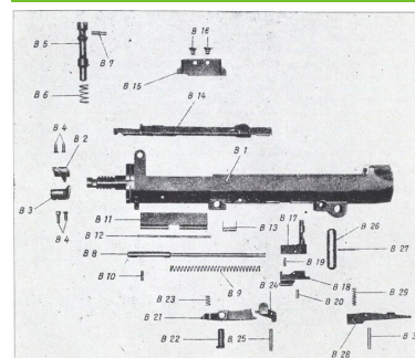
MG 34, Einzelteile: Gehäuse
