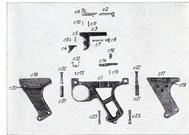
MG 34, Einzelteile: Griffstück
