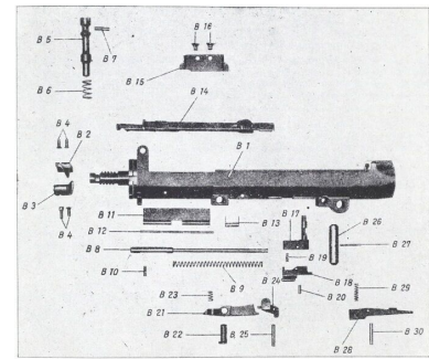
MG 34, Einzelteile: Gehäuse
