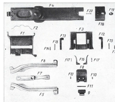
MG 34, Einzelteile: Zuführer und Zuführerdeckel
